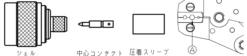
シェル 中心コンタクト 圧着スリーブ
