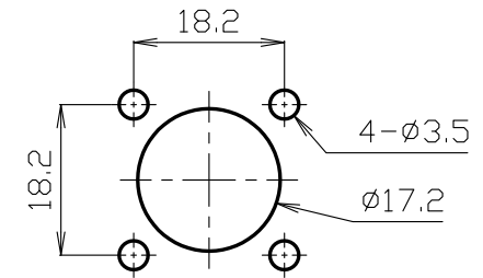
△ 取付穴参考寸法
