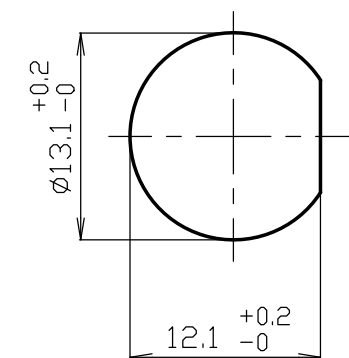
取り付け穴参考寸法
