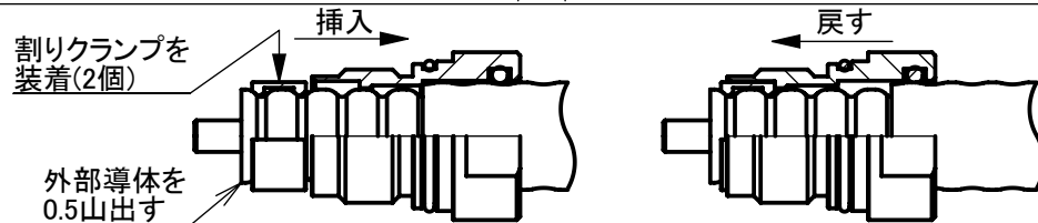
詳細図 B
