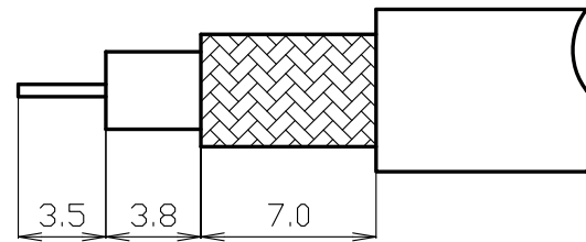
ケーブル取付図参考寸法
