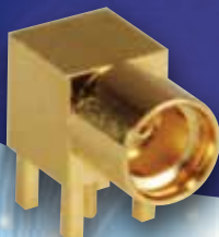
MMCX-LR-PCB 50Ω
